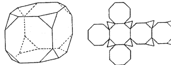
Cube tronqué :
