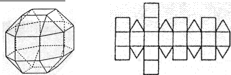
Rhombicuboctaèdre :
