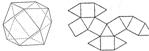
Cuboctaèdre :
