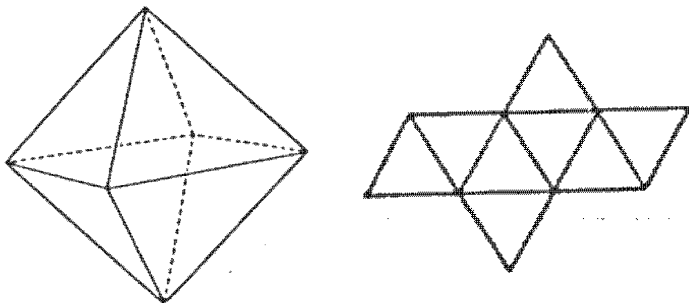
Octaèdre :
